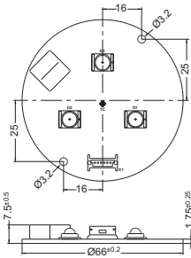
Triple Module
